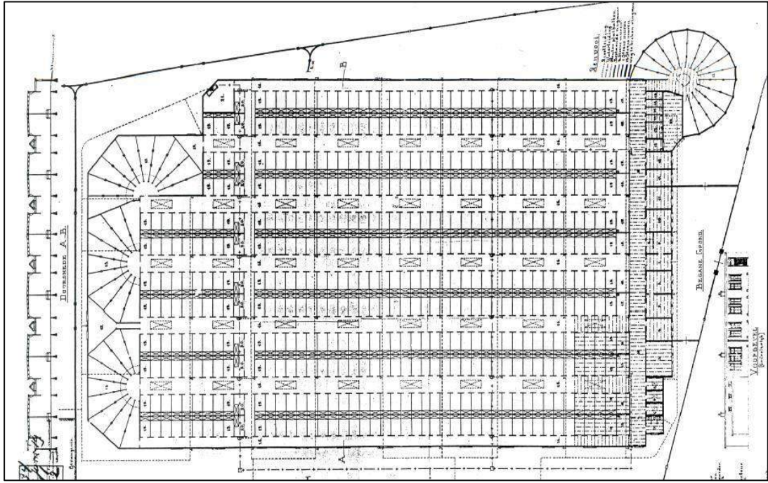
Plattegrond van de cellenbarak, gebouwd in 1919. (NMO)
