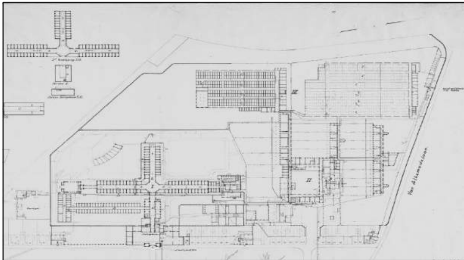
Plattegrond van het gevangeniscomplex anno 1952. I Strafgevangenis, II Bijzondere strafgevangenis, III Cellenbarakken. (NMO)
